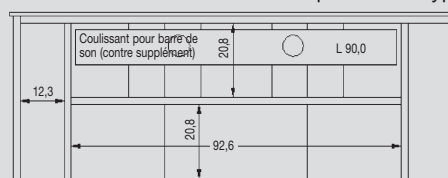
Dimensions intérieures des compartiments type 709
