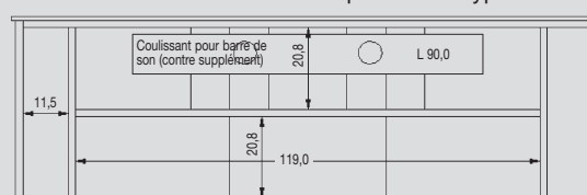
Dimensions intérieures des compartiments type 710
